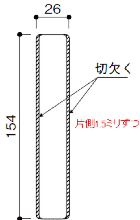
外召合せ框 内外化粧板取付用切欠き
